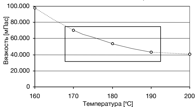
Показатели вязкости клея Иоватерм® 282.70/71
